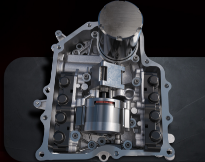
DSG Şanzıman Mekatronik İmaj Render
